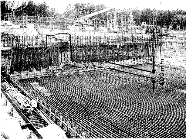
写真-13 打継ぎ位置の移動
