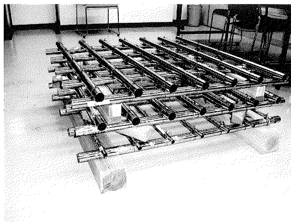
写真-10 配筋モデルを用いた打込み計画
