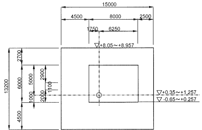
図-2 代表的な断面図 (5ブロック)
