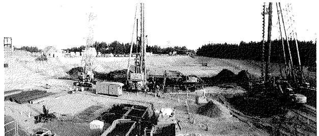
写真-3 SMW施工状況
