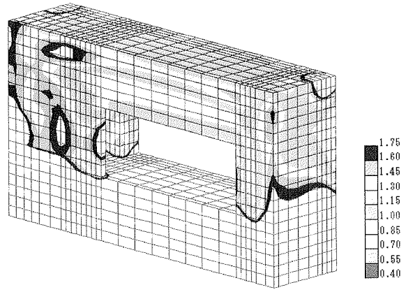
ひび割れ指数分布図
