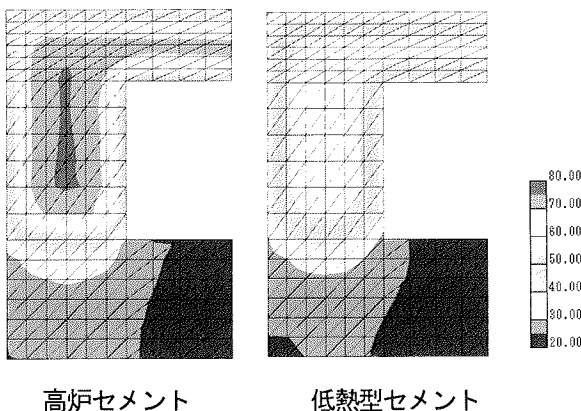
図-3 温度解析結果の例 (5 ブロック)
