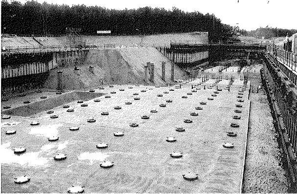
写真-4 均しコンクリート打設完了
