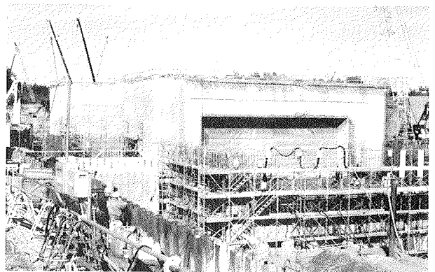
写真-8 対象構造物の施工状況 (型枠解体)
