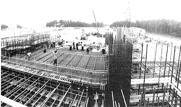
写真-5 頂版鉄筋組立状況 (9ブロック)
