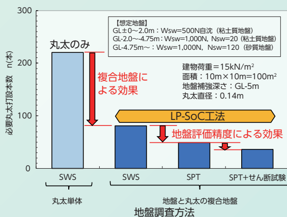
図-3 丸太打設本数削減効果
